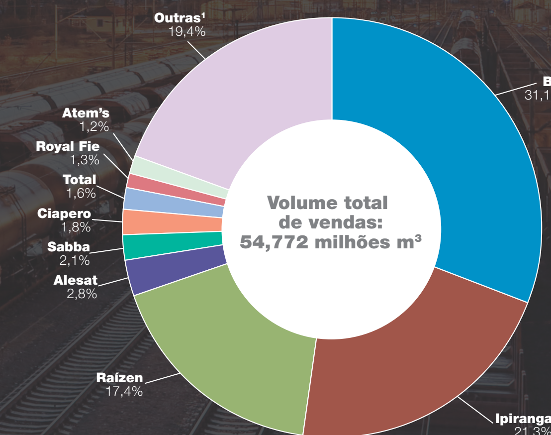
Gráfico 3.2 - Participação das distribuidoras nas vendas nacionais de óleo diesel - 2017
