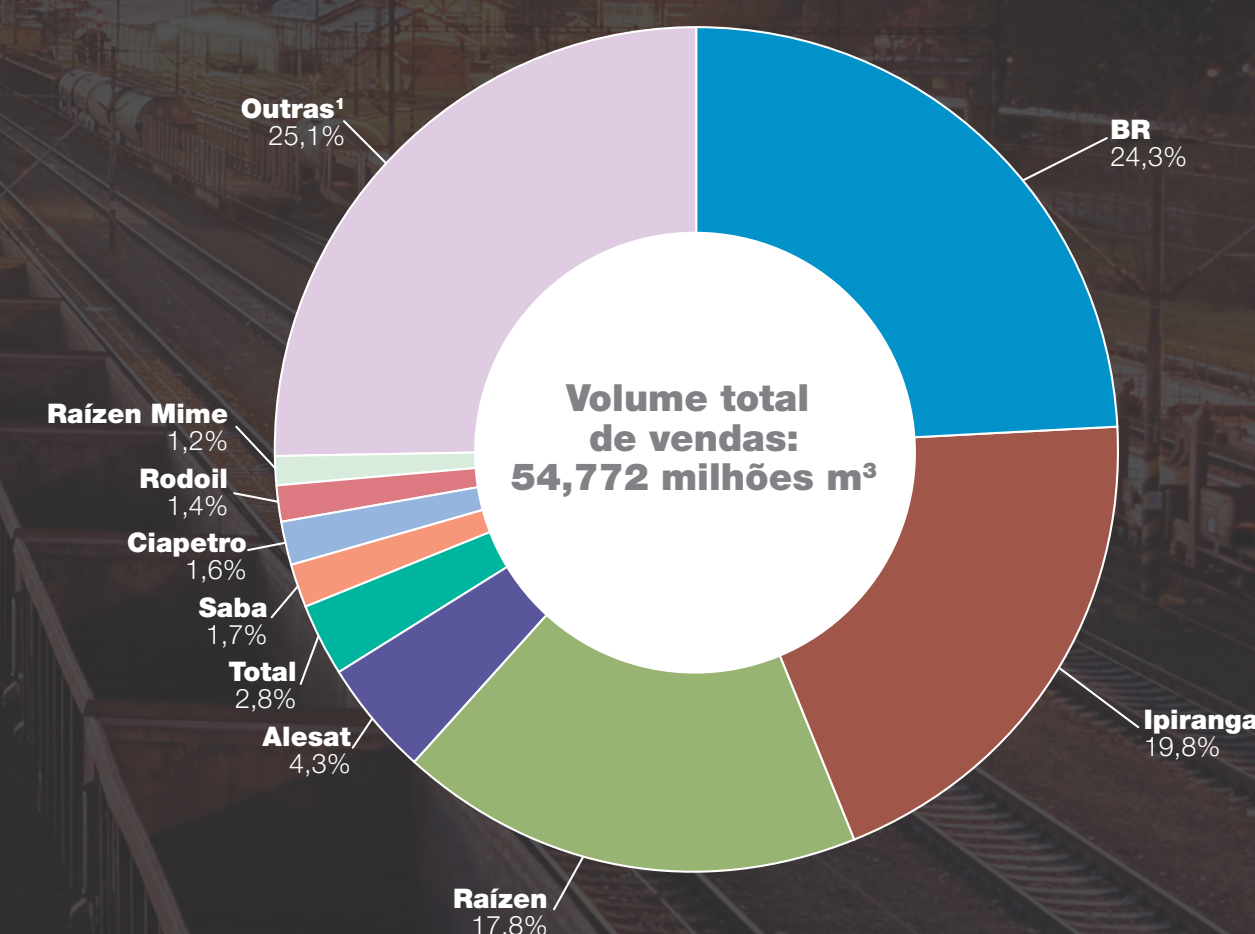
Gráfico 3.3 - Participação das distribuidoras nas vendas nacionais de gasolina C - 2017
